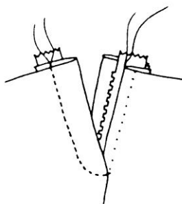
Zdrhovadlo všité do rozparku s podkrytem
