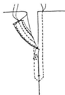
Připevnění tkanice zdrhovadla na švovou záložku
